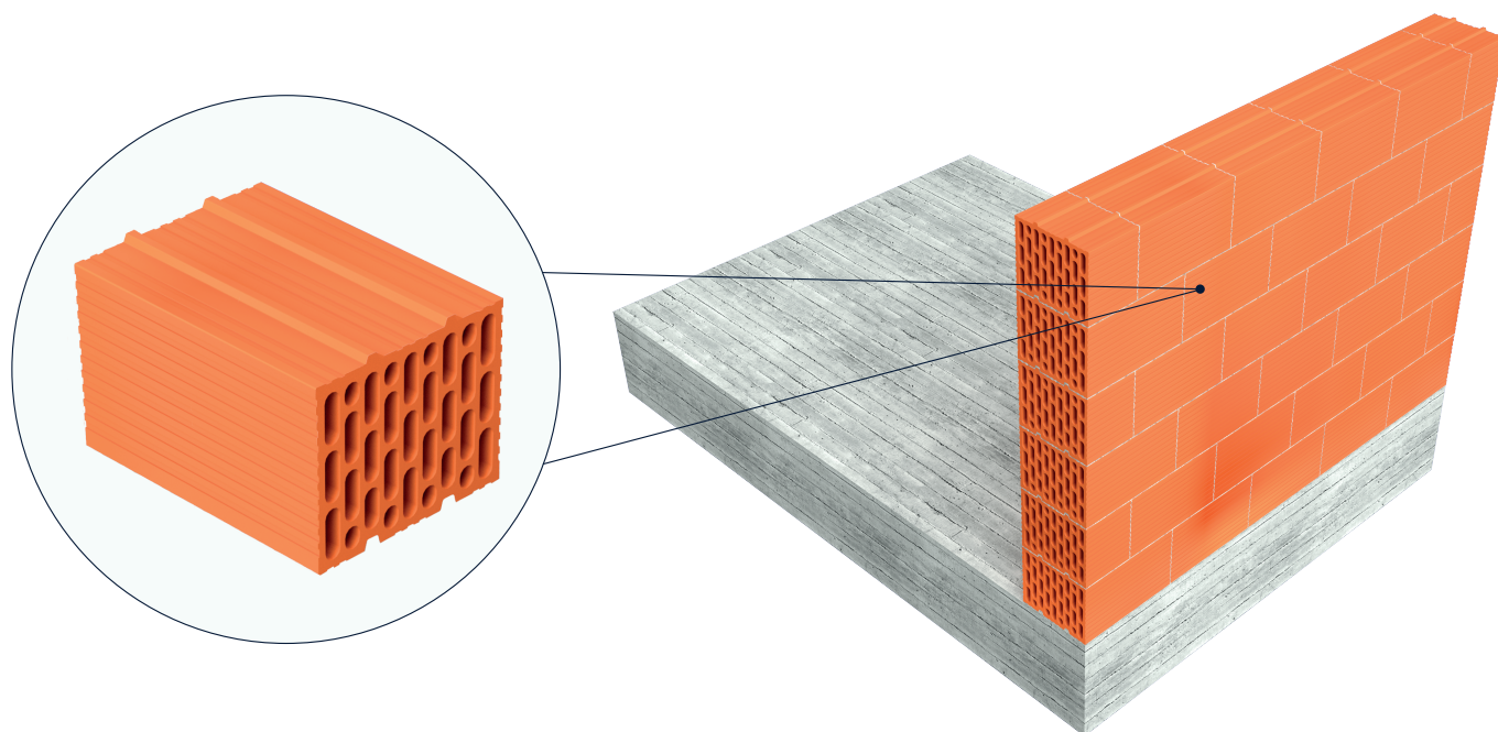
MUESTRA DE PETO ELABORADO CON LADRILLO ALIGERADO GRAN FORMATO “SATEPAS 24”
