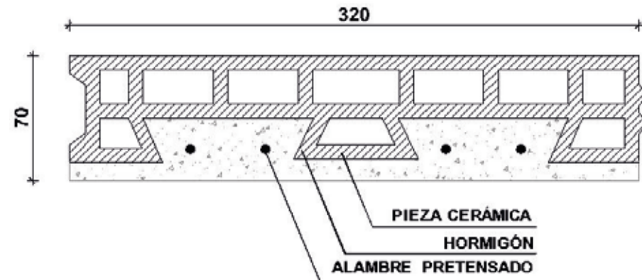
SECCIÓN TRANSVERSAL COTAS EN mm.
